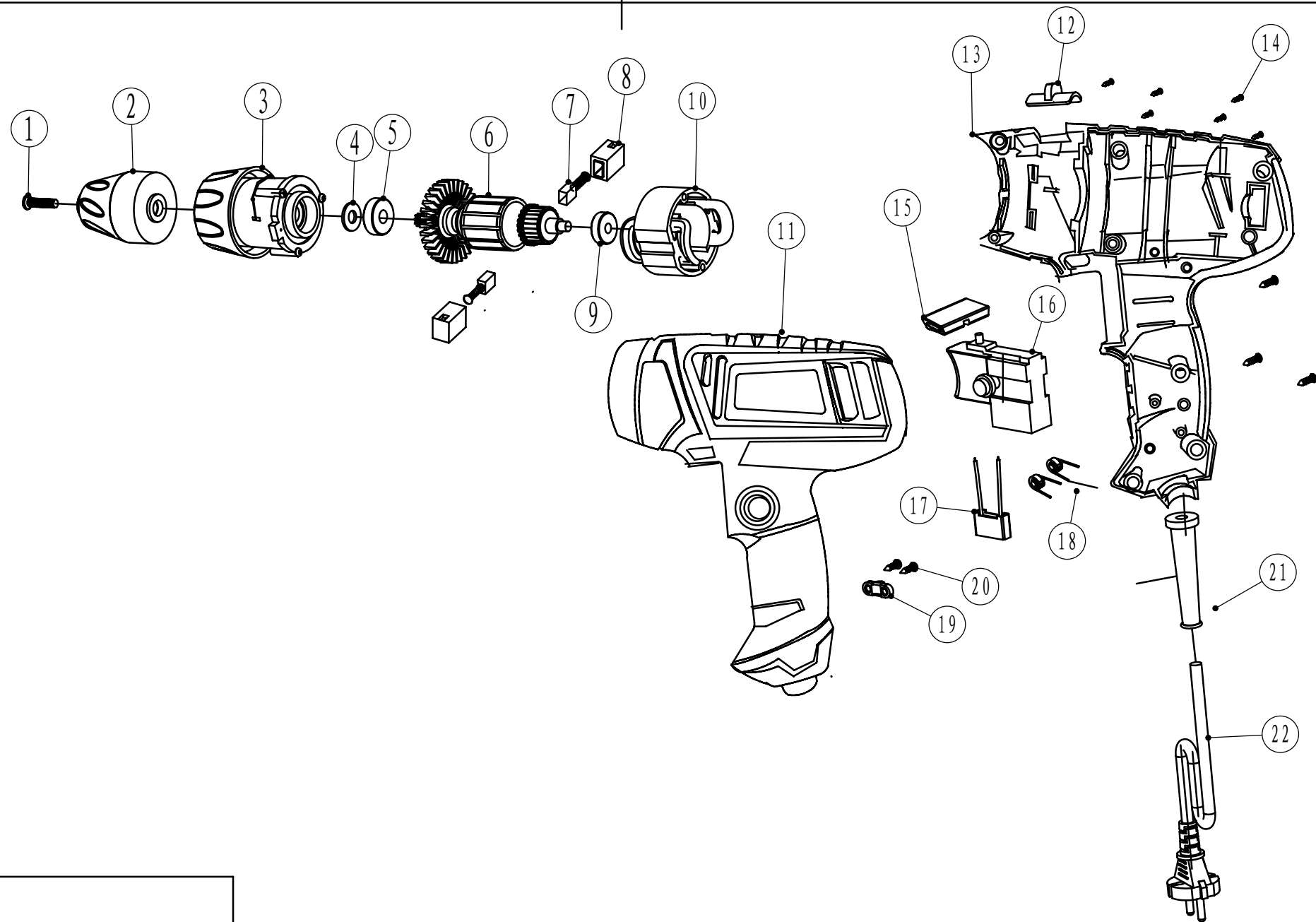
6109-2爆炸图
